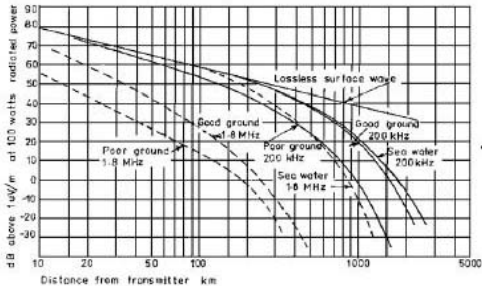
Fig. 9 Ricevibilità del segnale in funzione della frequenza e della distanza del trasmettitore
