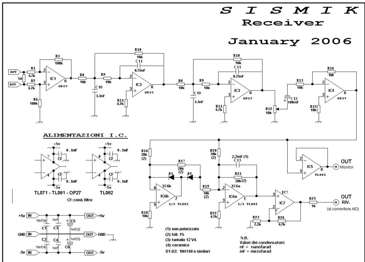
Fig. 28 Schema modificato del ricevitore Prediktör con banda passante da 0 a 24 kHz
