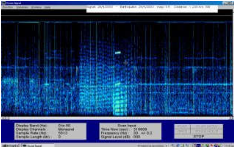
Fig.31 Possibile candidato di evento precursore sismico registrato a Atene da Dionysios Dimakos (SV1ZJ) - Evento del 29.4.2003, Magnitudo 5 Richter a circa 230 km SW di distanza.
