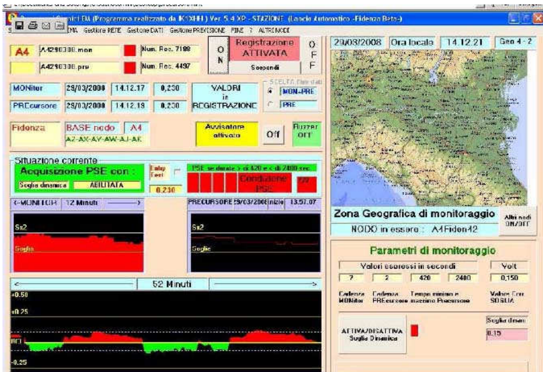
Fig. 26 Presunto precursore sismico della scossa verificatasi il 29 Marzo 2008 con epicentro nell'Appennino tosco-emiliano alle 18:19 UTC, con magnitudo 2,5 e profondità pari a 18 Km.
