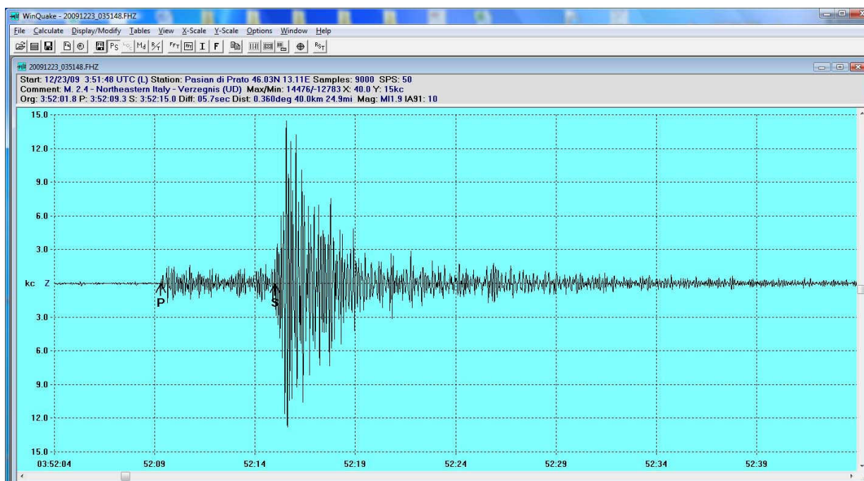
Fig. 32 Esempio di analisi di un tracciato sismico con il programma Winquake (Shareware)
