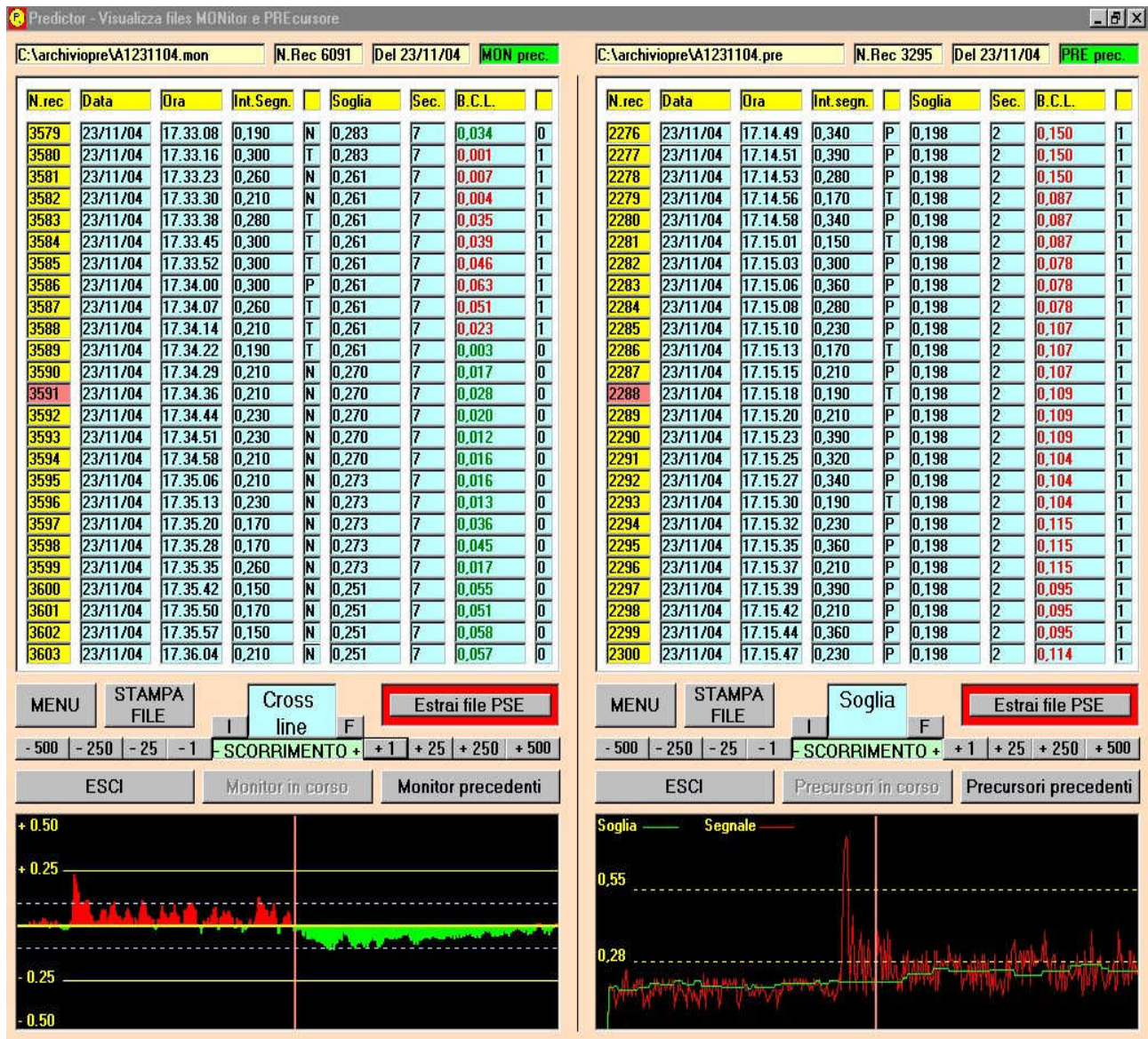
Fig. 23 Un possibile precursore rilevato in data 23/11/04 alle ore 17 circa (alle ore 23.59 dello stesso giorno si ebbe un evento sismico nella zona di Brescia con intensità di oltre il 5 grado della scala Richter)
