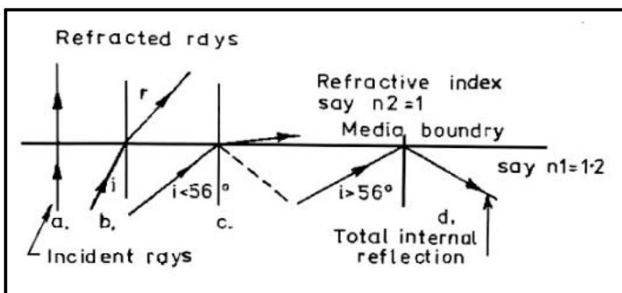
Fig. 6 Schema esempi di riflessione e rifrazione delle onde elettromagnetiche
