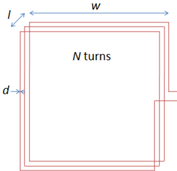
Fig. 16 Schema di un'antenna a loop su telaio di forma quadrata dove: W è la larghezza del lato del telaio, l è la lunghezza dell'avvolgimento d è il diametro del filo conduttore N turns è il numero delle spire.
