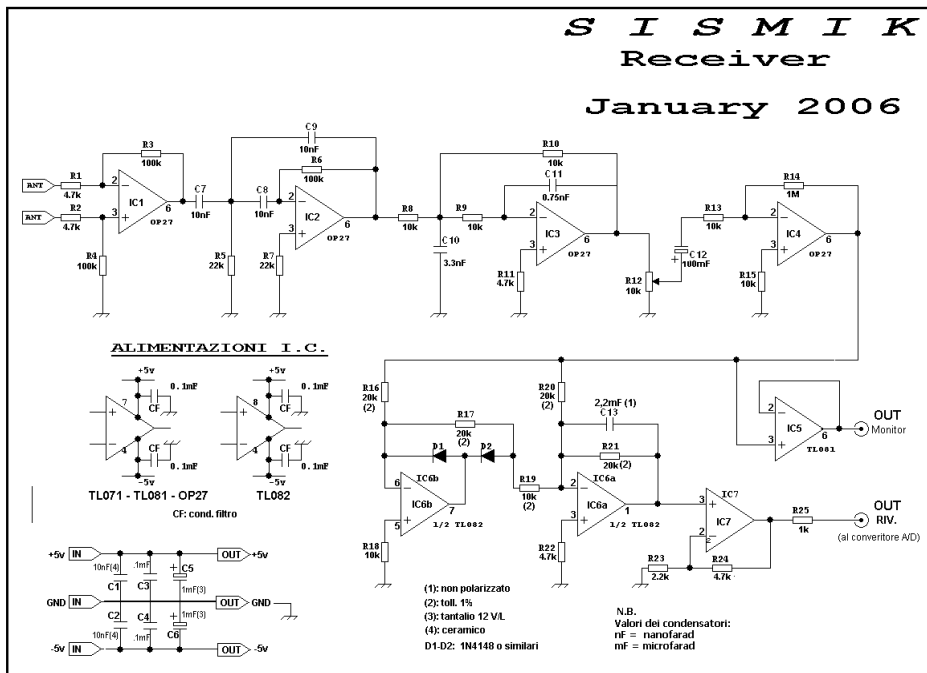
Fig. 19 Schema elettrico ricevitore del sistema Prediktor
