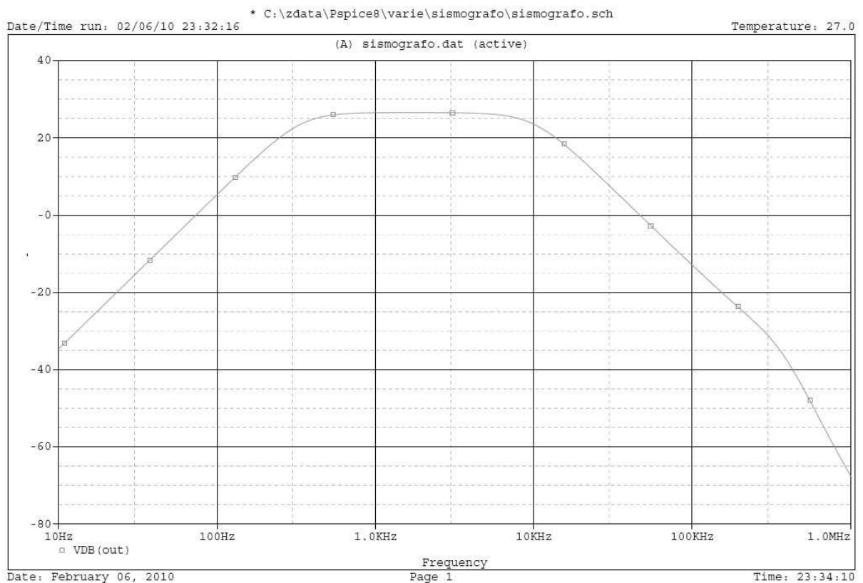
Fig. 20 Banda di frequenze passante nel ricevitore del sistema Prediktor: da 300 Hz a 10 kHz
