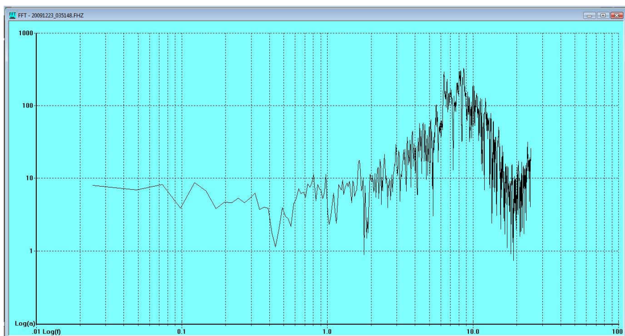
Fig. 33 Esempio di analisi dello spettro di un tracciato sismico con il programma Winquake (Shareware)
