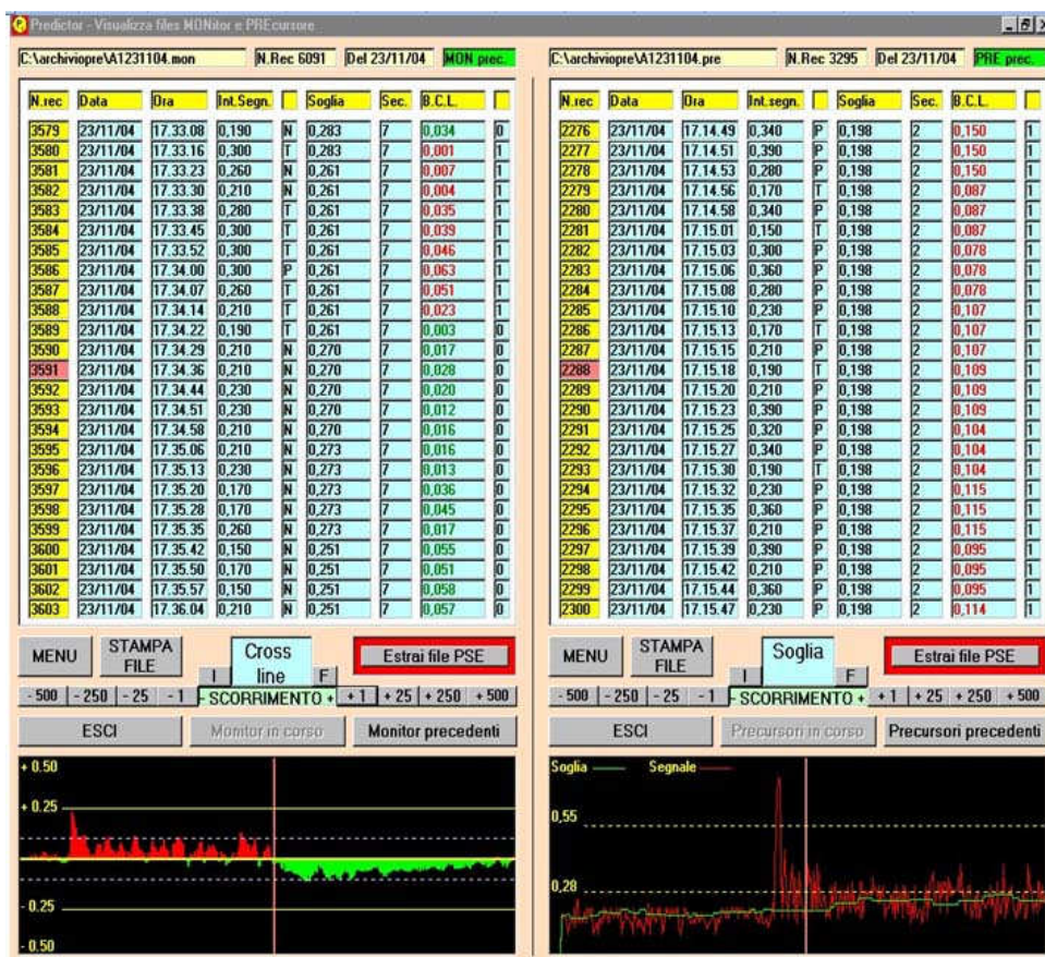
Fig. 27 Un probabile precursore rilevato in data 23/11/04 alle ore 17 circa dalla stazione di Sarzana (SP) (alle ore 23.59 dello stesso giorno si ebbe l'evento sismico della zona di Brescia con intensità di oltre il 5 grado della scala Richter).
