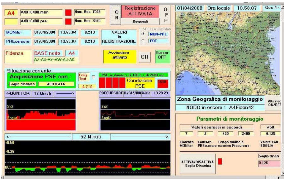
Fig. 25 Presunto precursore sismico della scossa verificatasi il 1 Aprile 2008 ore 19:43 UTC con epicentro nelle alpi Marittime: di magnitudo ML 2.3 e profondità 10 km
