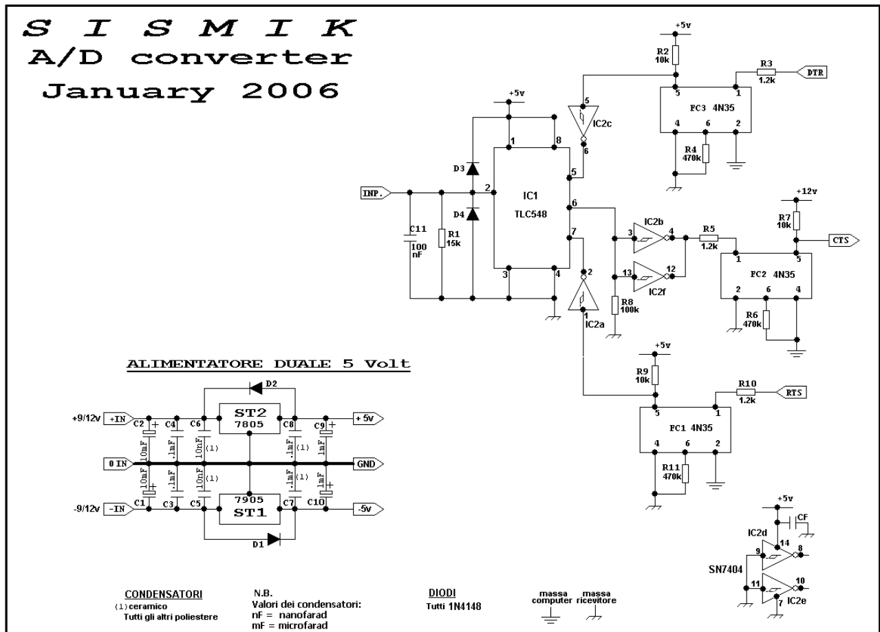
Fig. 21 Schema elettrico del convertitore A/D del sistema Prediktor
